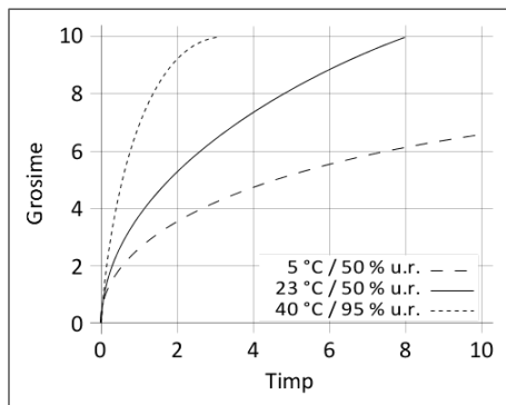
Diagrama 1: Viteza de întărire pentru Sikasil® WS-305 EU
