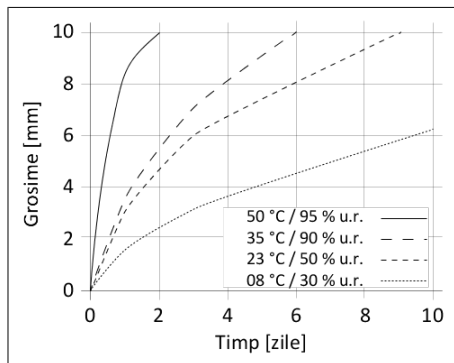
Diagrama 1. Viteza de întărire pentru Sikasil® SG-20
